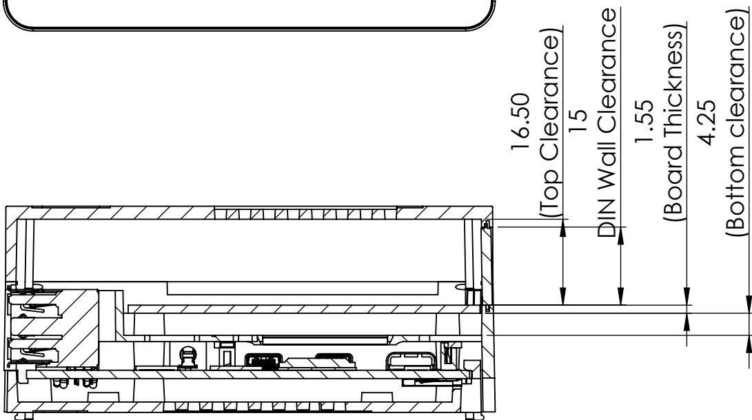
SECTION A-A
